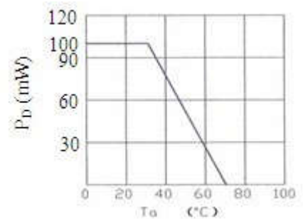
温度与功耗
