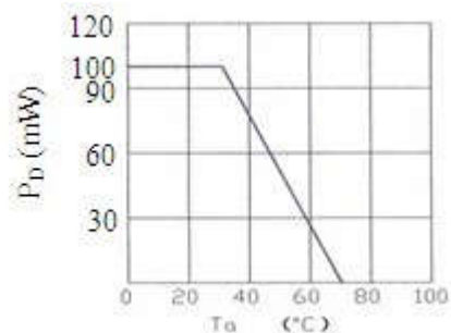
温度与功耗
