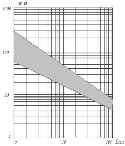
图 3 GM4537-1
