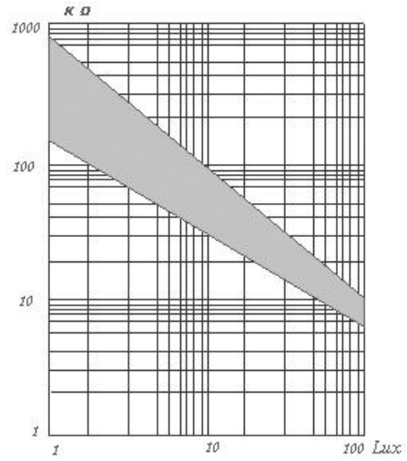
图 4 GM4537-2
