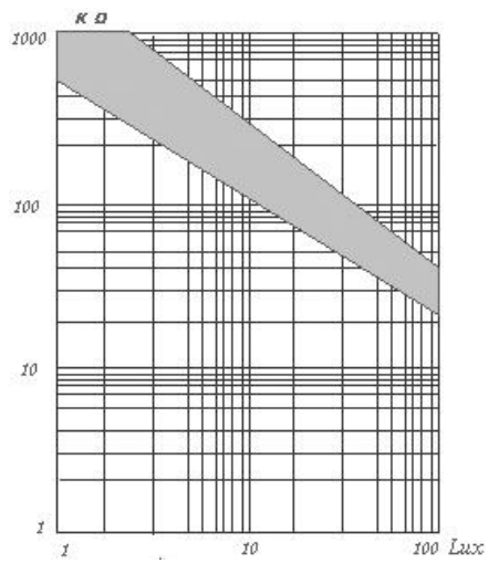
图 4 GM4537-2
